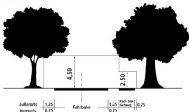
Lichtraumprofil
